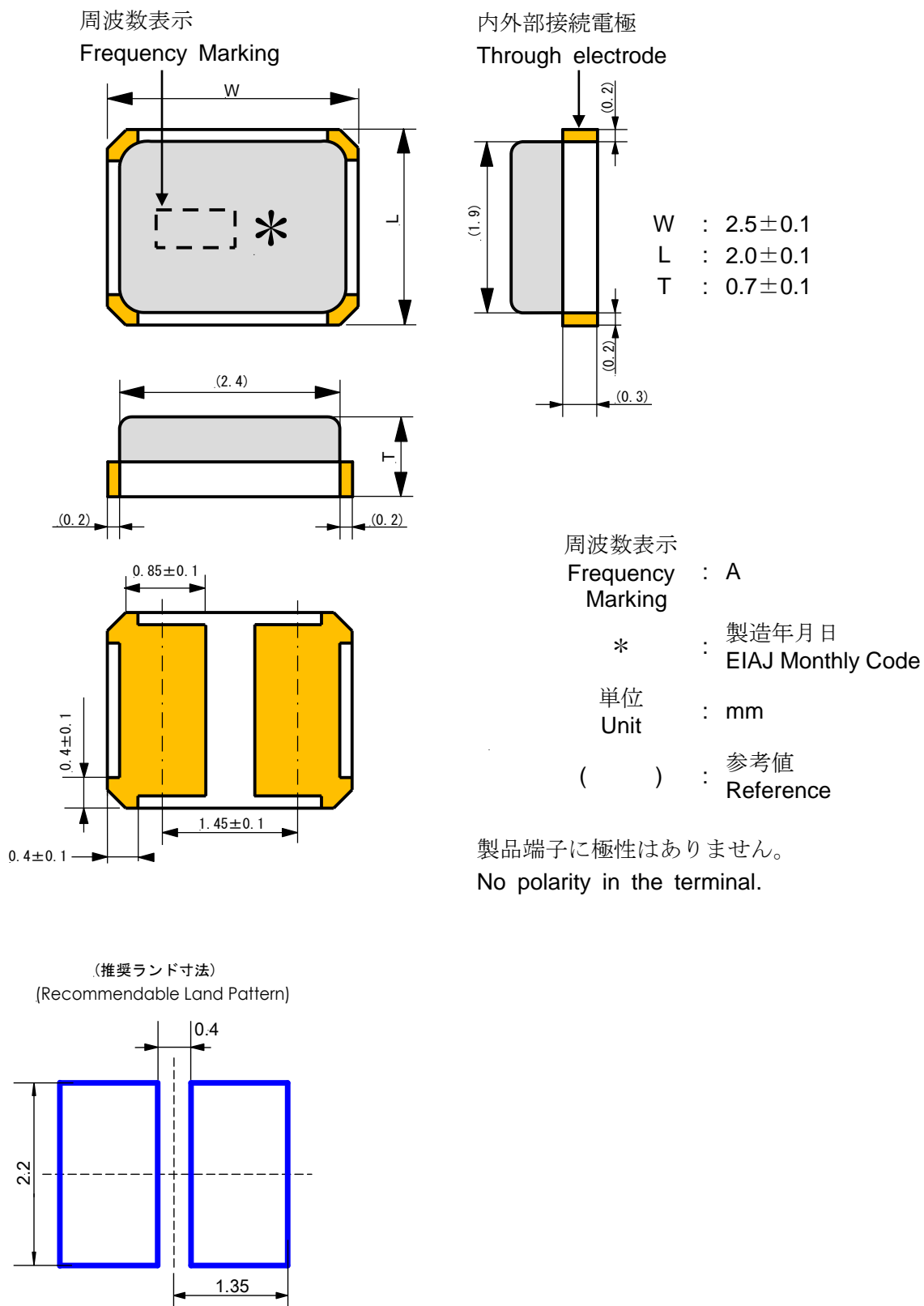
第1図 外形寸法図 Figure 1. Dimensions
